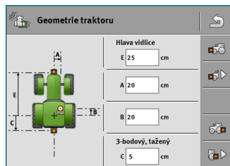
Příkladná geometrie traktoru
