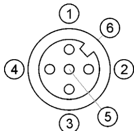
Zdiřka M12: Kamera
