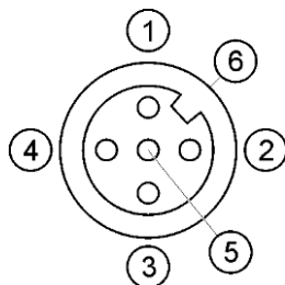
Zdířka M12: Ethernet
