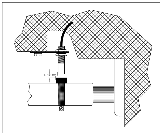
Obr. 5-1 Snímač X na kloubové hřídeli
