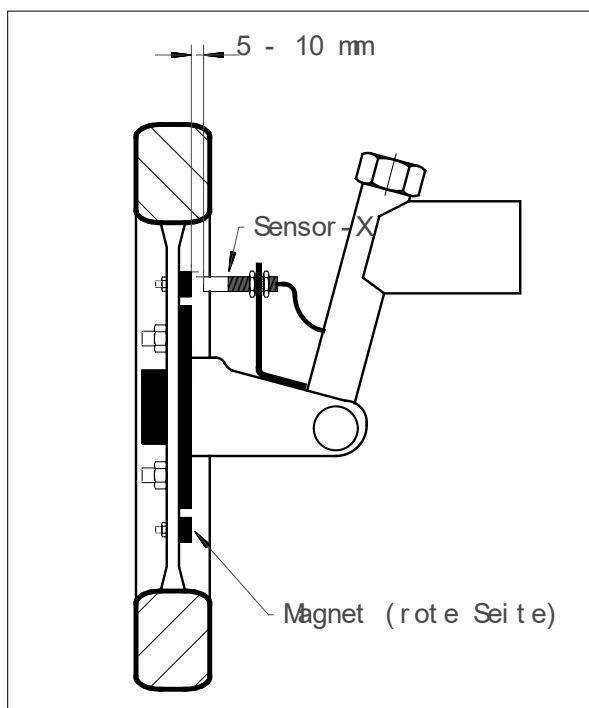
Obr. 5-2 Snímač X na kole traktoru
