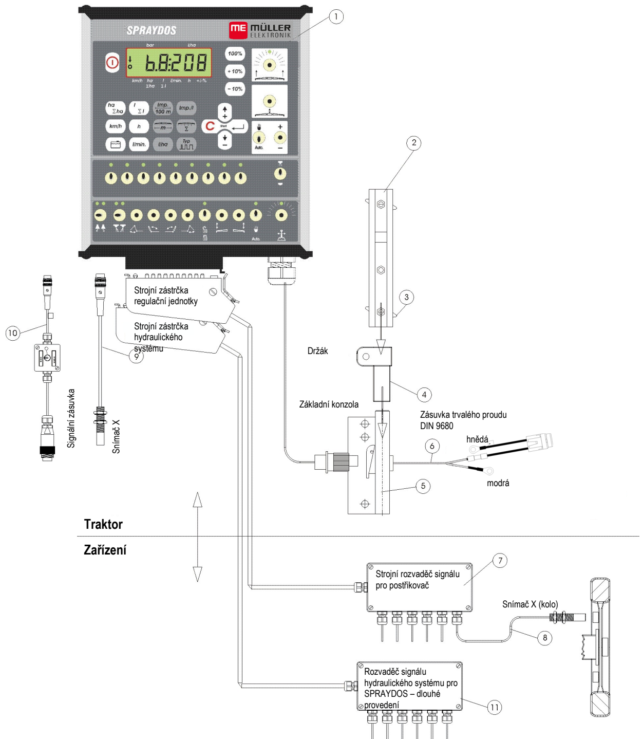
Obr. 4-1 Přehled SPRAYDOS
